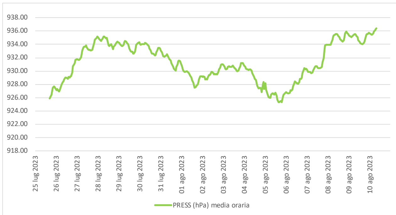
Figura 6.3 - Pressione atmosferica.
